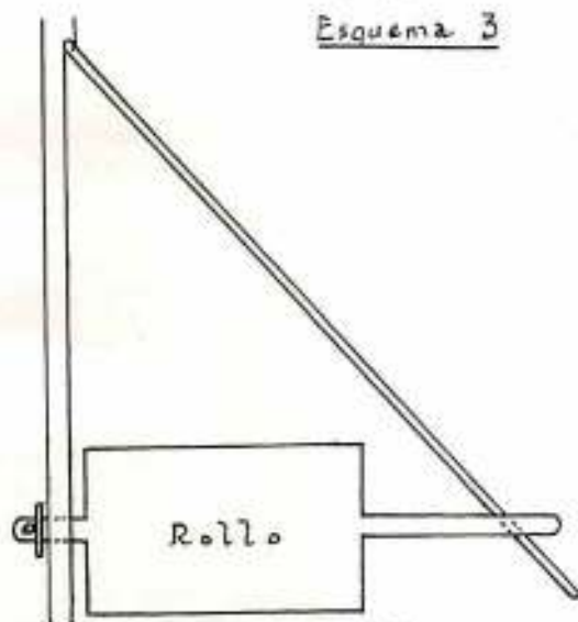
EMPATE DEL EJE DEL ROLLO EN EL MAYAL Vista lateral
