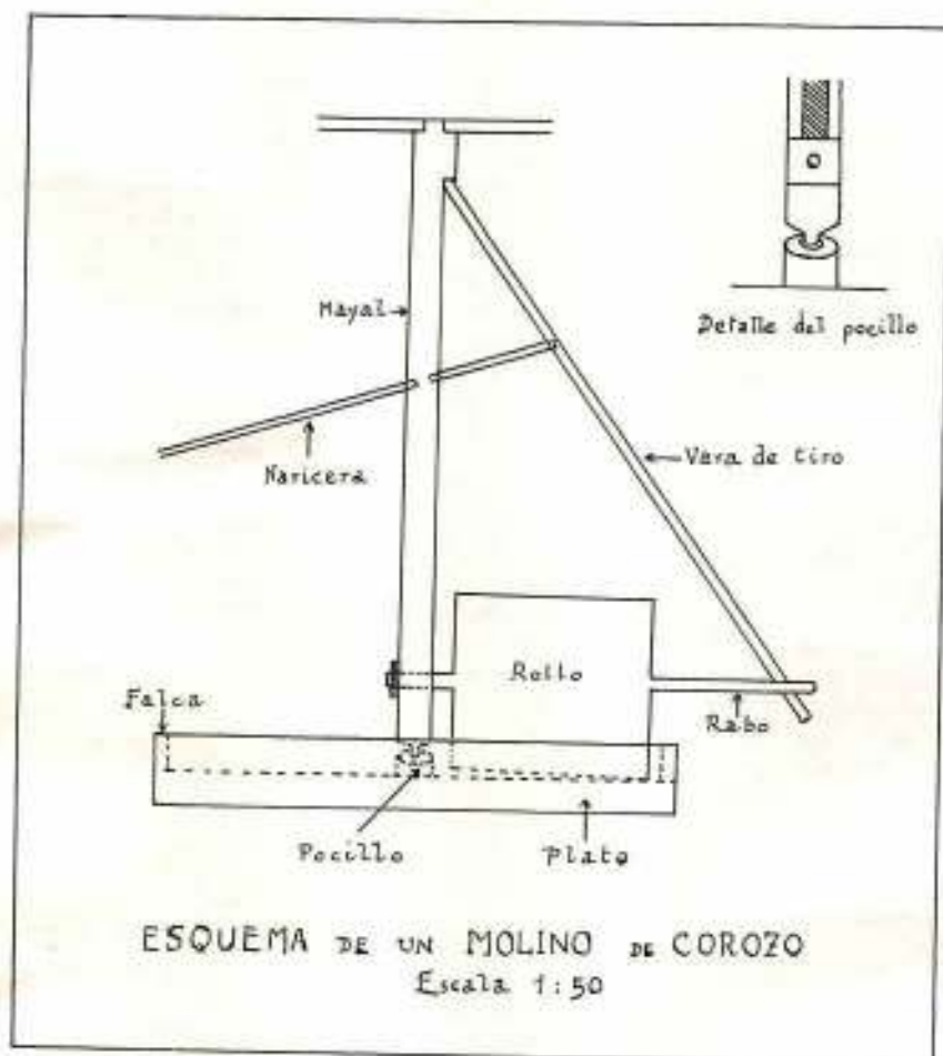
Dibujo Nº 8. Esquema de un molino de corozo. Original del autor. Véase descripción detallada en la página 80.
