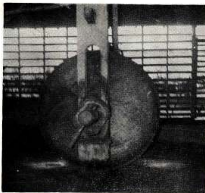
Foto N° 22. Detalle que muestra la manera como se ajusta el eje del rolo al mayal Molino "Flor de María".
